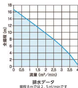
ポンプ SDH200AK
